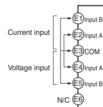
Linear Sensor Indicator K3HB-S
